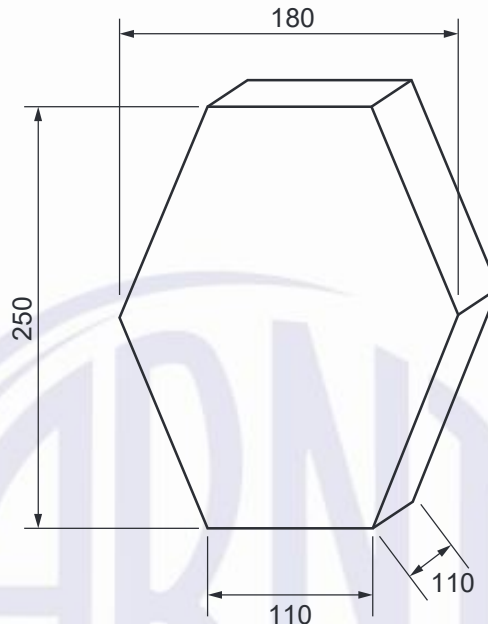
Figura 6 – Gabarito prismático
