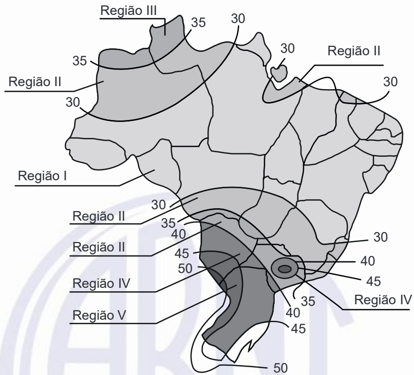
Figura E.2 – Exemplo de análise do gráfico de isopletas em relação à velocidade do vento
