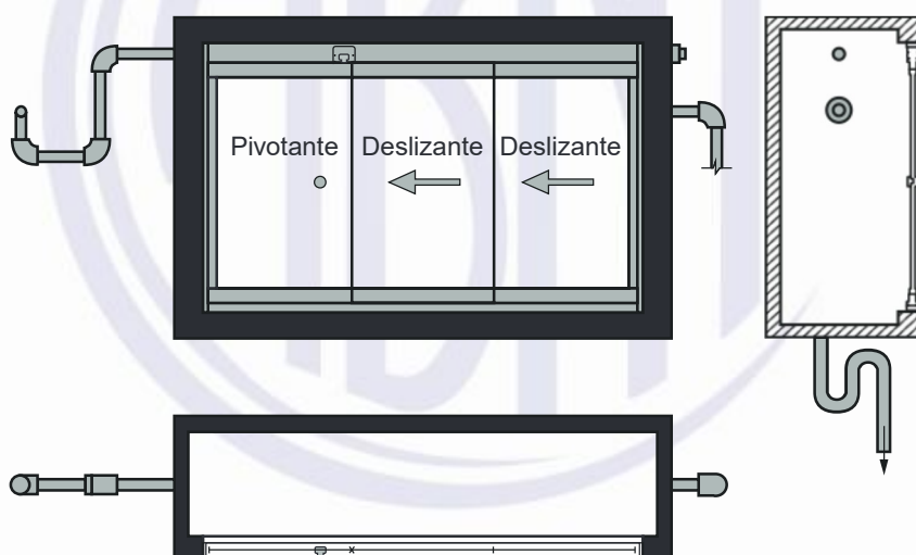
Figura A.1 – Vista esquemática de um modelo de câmara de ensaio
