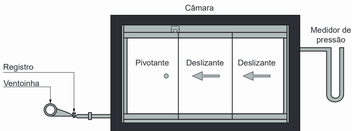
Figura A.2 – Esquema geral de um modelo de sistema de pressurização
