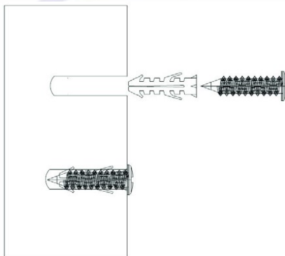
Figura 4 – Demonstrativo de fixação do parafuso na alvenaria
