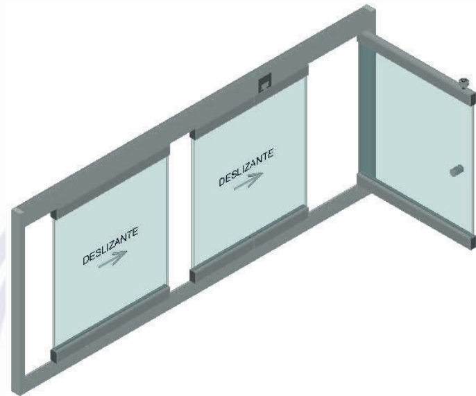
Figura 2 – Exemplo de tipologia com abertura total
